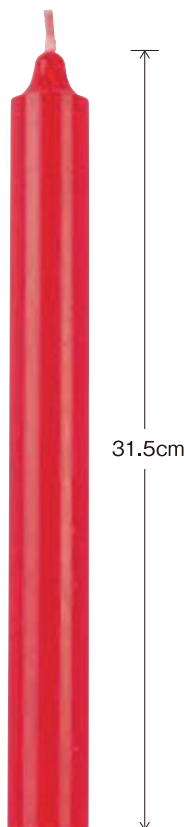
238 AF062R 大ローソク60号 (赤) 寸 法: \phi 33 \times H315\text{mm} 入 数: 60本 (バラ詰) 燃焼時間: 約22時間
