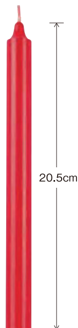
236 AF107R 大ローソク10号 (赤) 12本 寸 法: \phi 17 \times H205\text{mm} 入 数: 30函 燃焼時間: 約5時間
